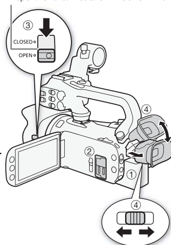
Переключатель заслонки объектива
